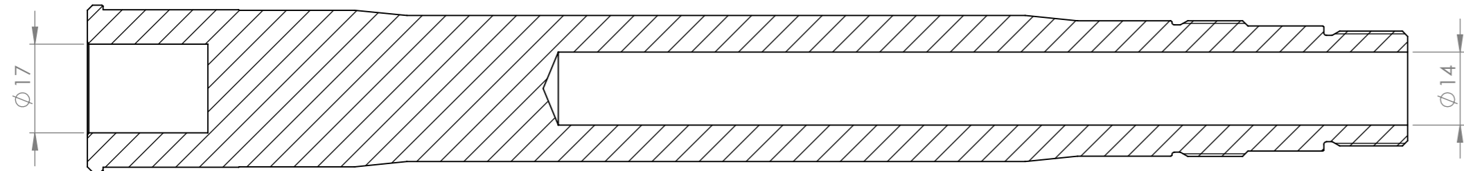
SCHNITT A-A
