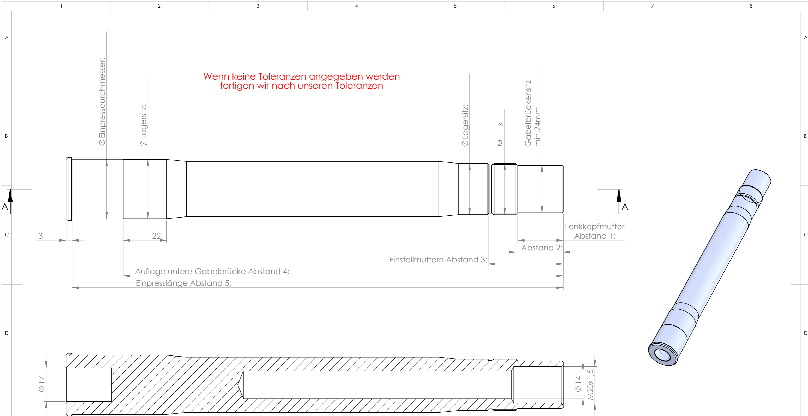
SCHNITT A-A
